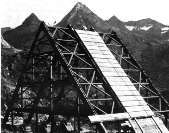
Situación de las obras de construcción del refugio de Piedrafita.
